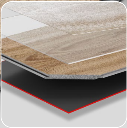
zintegrowany podkład podkład XPO o grubości 1 mm ; odporność na obciążenia CS > 400 kPa
